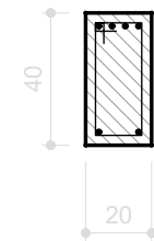
SEÇÃO A-A ESC 1:25
